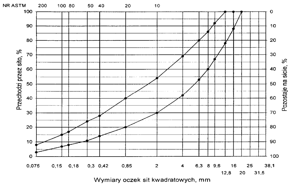
Rys. 9. Krzywe graniczne uziarnienia mieszanki mineralnej BA od 0 do 16 mm do warstwy wyrównawczej nawierzchni drogi o obciążeniu ruchem KR1 lub KR2
