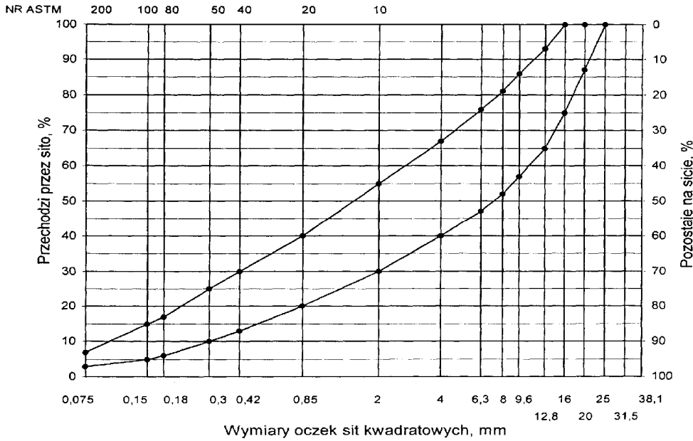
Rys. 8. Krzywe graniczne uziarnienia mieszanki mineralnej BA od 0 do 20 mm do warstwy wyrównawczej nawierzchni drogi o obciążeniu ruchem KR1 lub KR2
