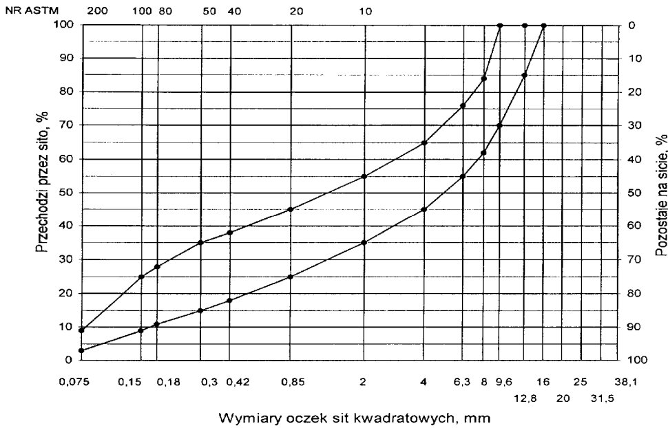
Rys. 10. Krzywe graniczne uziarnienia mieszanki mineralnej BA od 0 do 12,8 mm do warstwy wyrównawczej nawierzchni drogi o obciążeniu ruchem KR1 lub KR2
