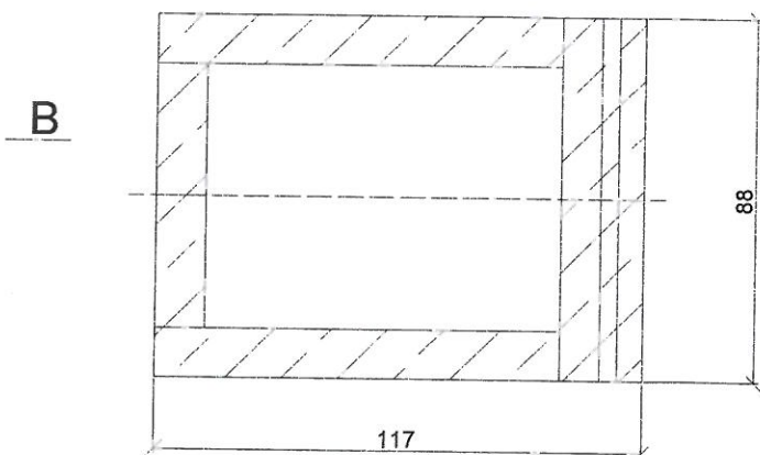
Rzut wylotu rury kanalizacyjnej
