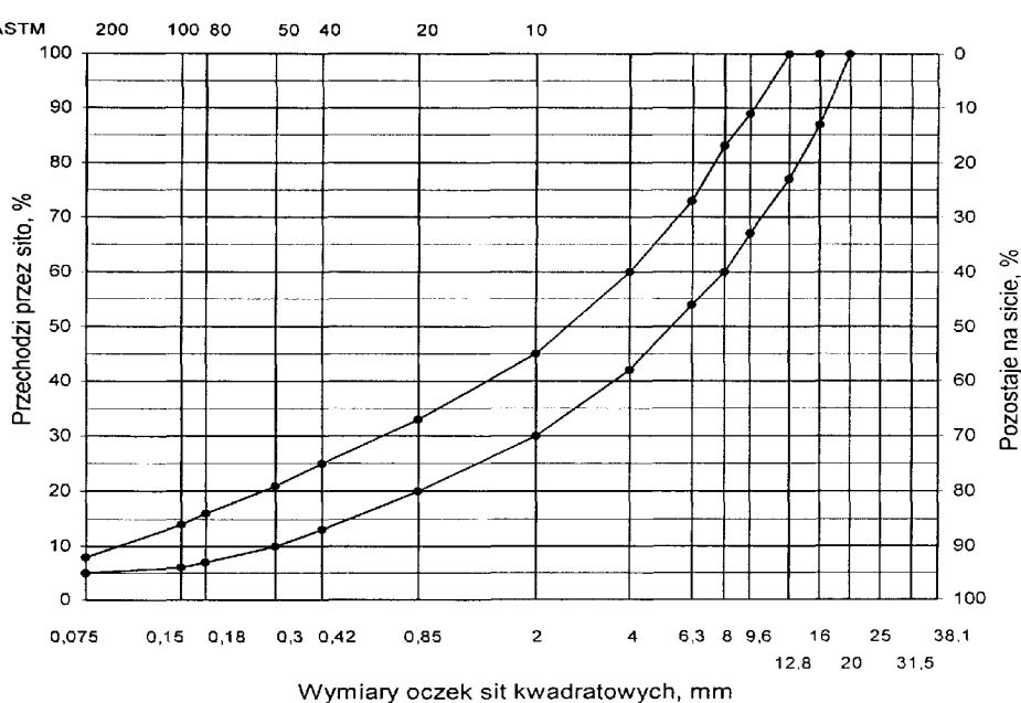
Wymagania wobec mieszanek mineralno-asfaltowych i warstwy wiążącej, wyrównawczej oraz wzmacniającej z betonu asfaltowego
