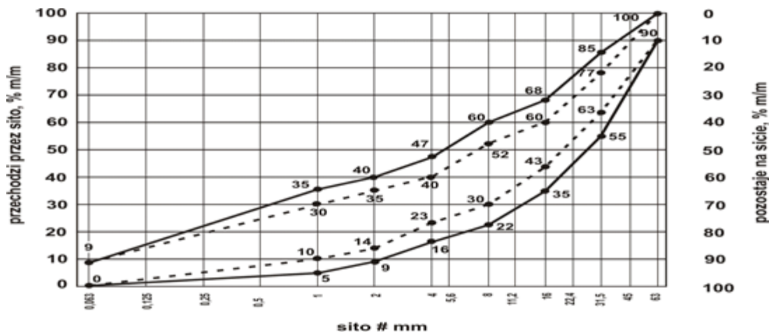
Rys. 3 Uziarnienie mieszanki 0/63
