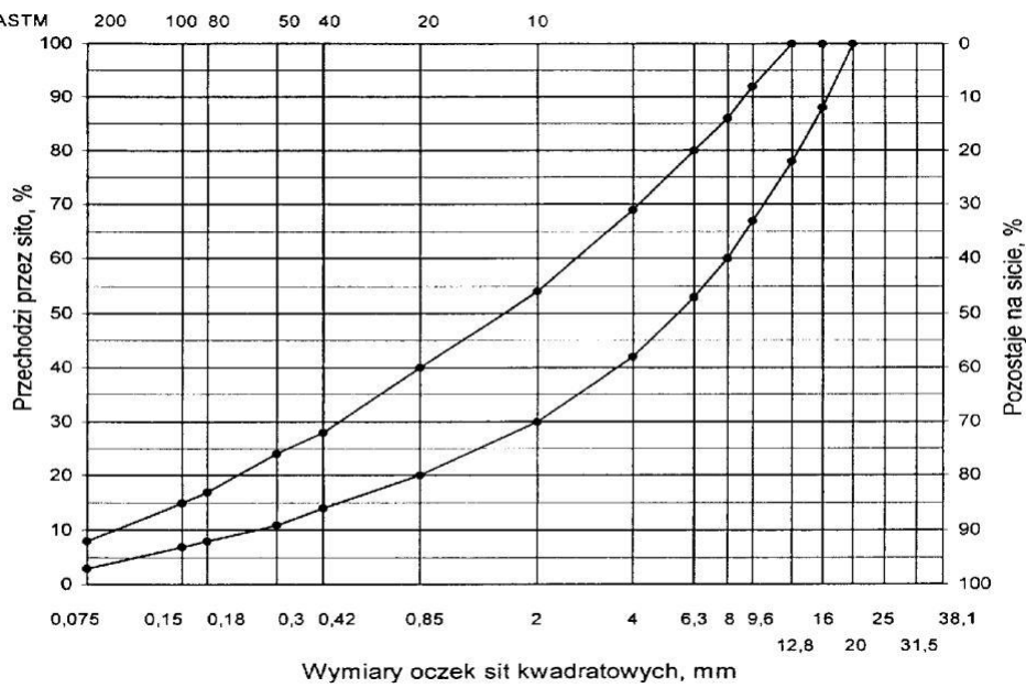
wyrównawczej i wzmacniającej nawierzchni drogi o obciążeniu ruchem KR1 lub KR2
