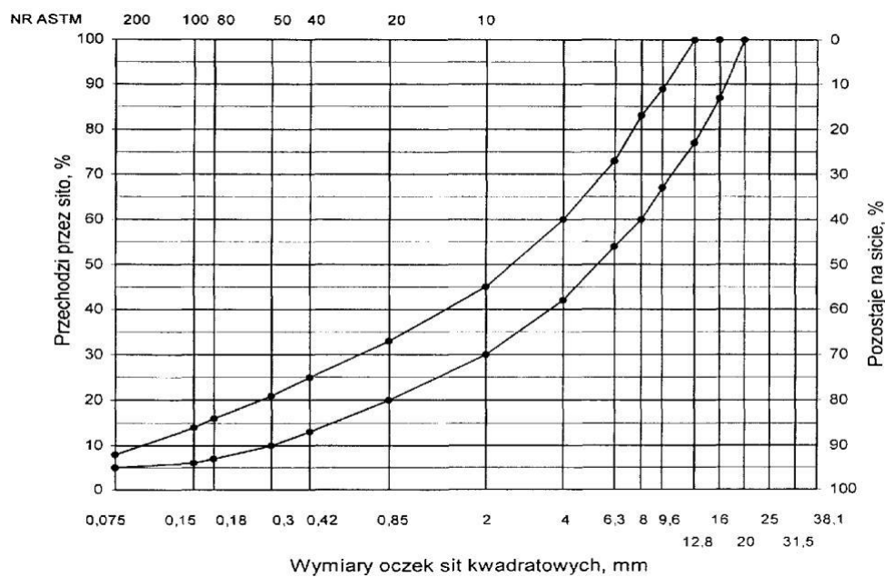
12. Krzywe graniczne uziarnienia mieszanki mineralnej BA od 0 do 20 mm do warstwy wiążącej, wyrównawczej i wzmacniającej nawierzchni drogi o obciążeniu ruchem od KR3 do KR6
