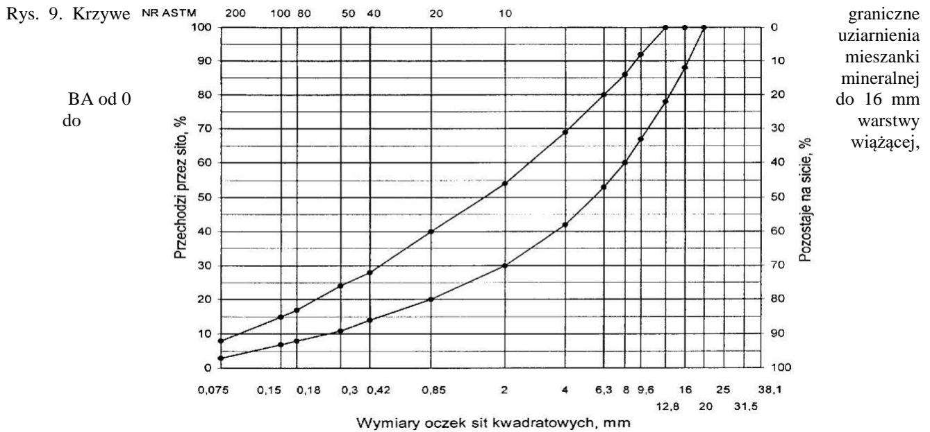
Rys. 9. Krzywe graniczne uziarnienia mieszanki mineralnej BA od 0 do 16 mm warstwy wiążącej, wyrównawczej i wzmacniającej nawierzchni drogi o obciążeniu ruchem KR1 lub KR2
