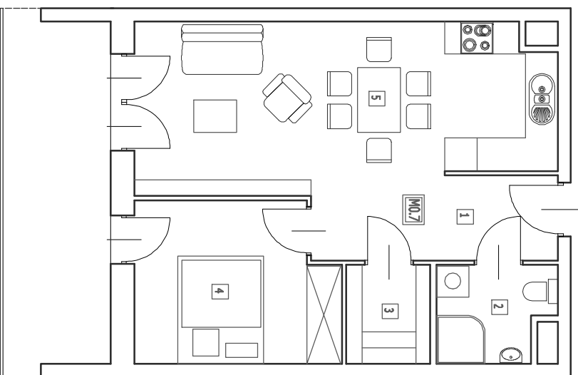
RZUT LOKALU
