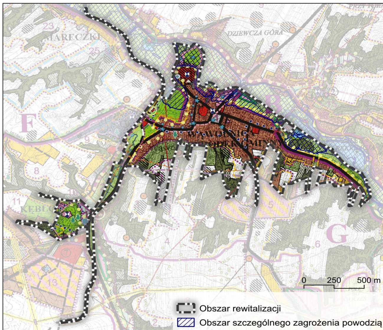
Rysunek 4 Wyrys ze Studium uwarunkowań i kierunków zagospodarowania przestrzennego dla obszaru rewitalizacji m. Wąwolnica
